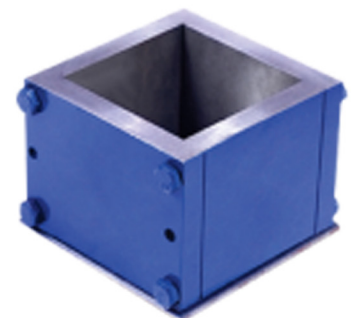
Cube Mould 7.06cm X 7.06cm
